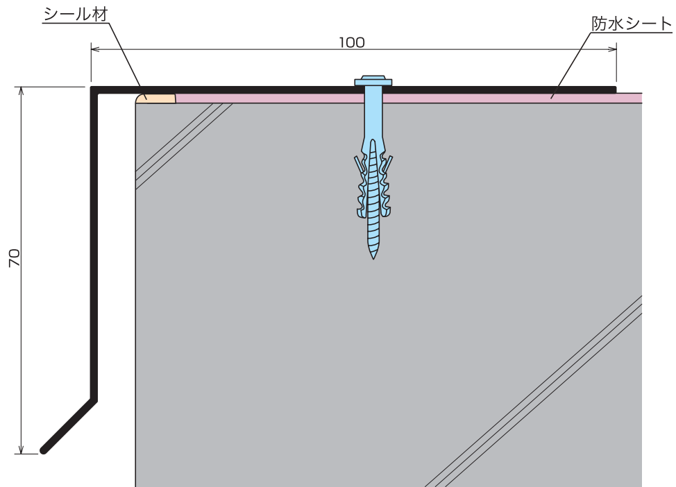
TA-107納まり図
