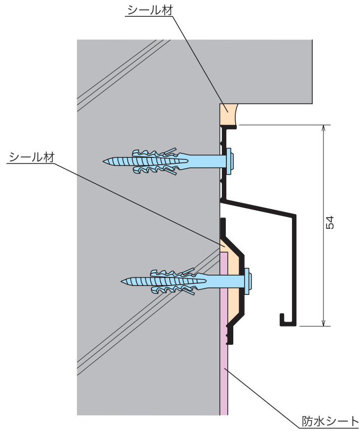
TA-206納まり図
