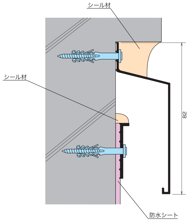
TA-208納まり図
