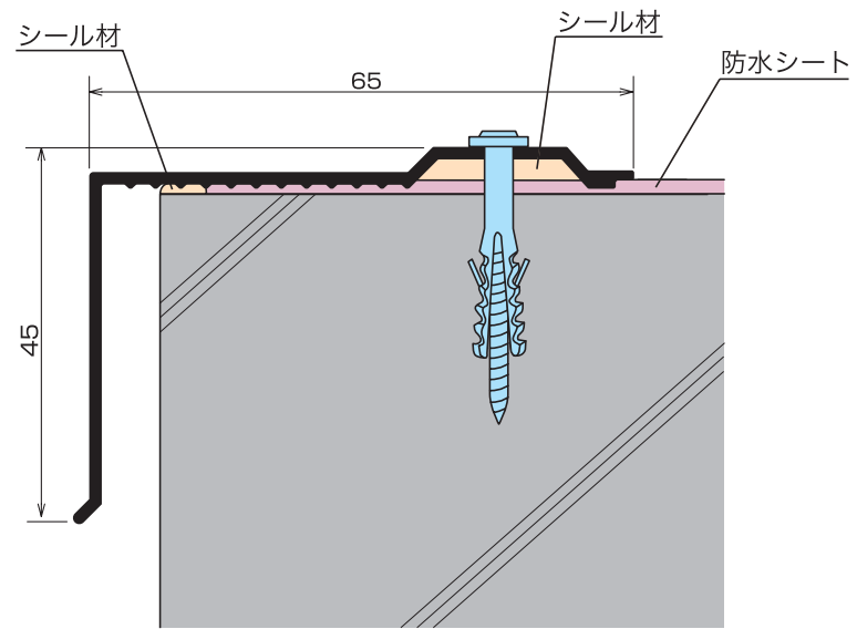
TA-46納まり図
