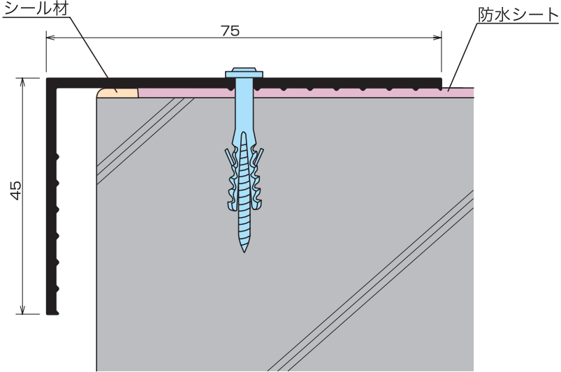
TA-79納まり図
