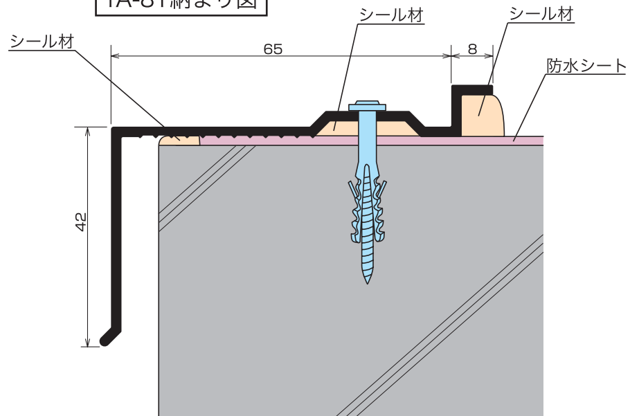
TA-81納まり図
