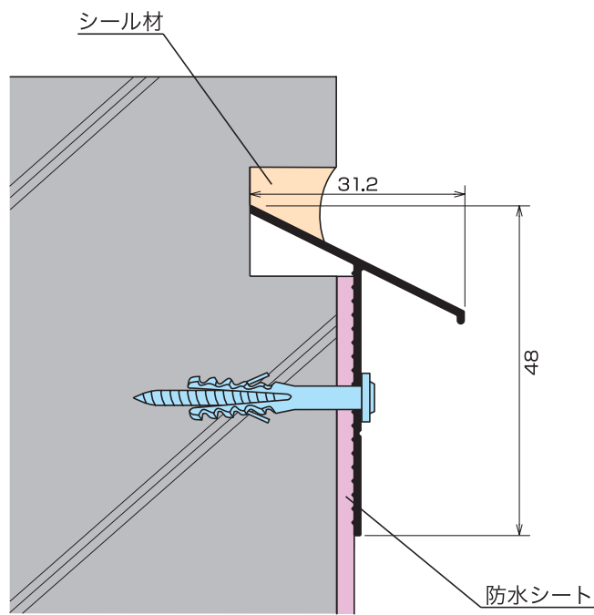
T-16納まり図
