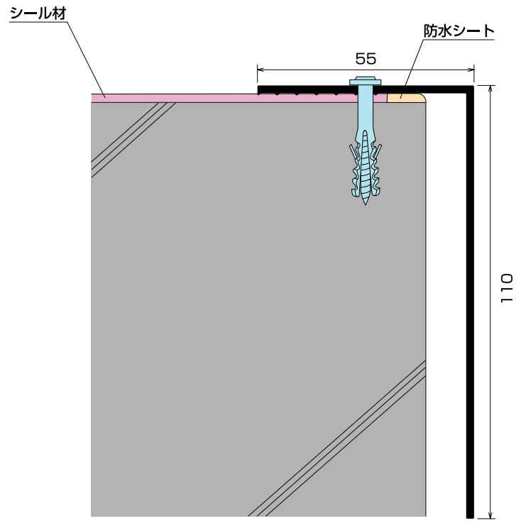
TA-115納まり図
