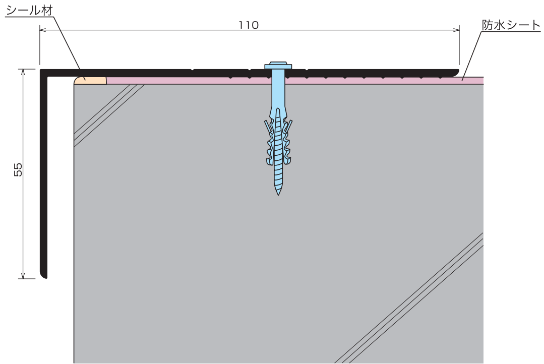
TA-117納まり図
