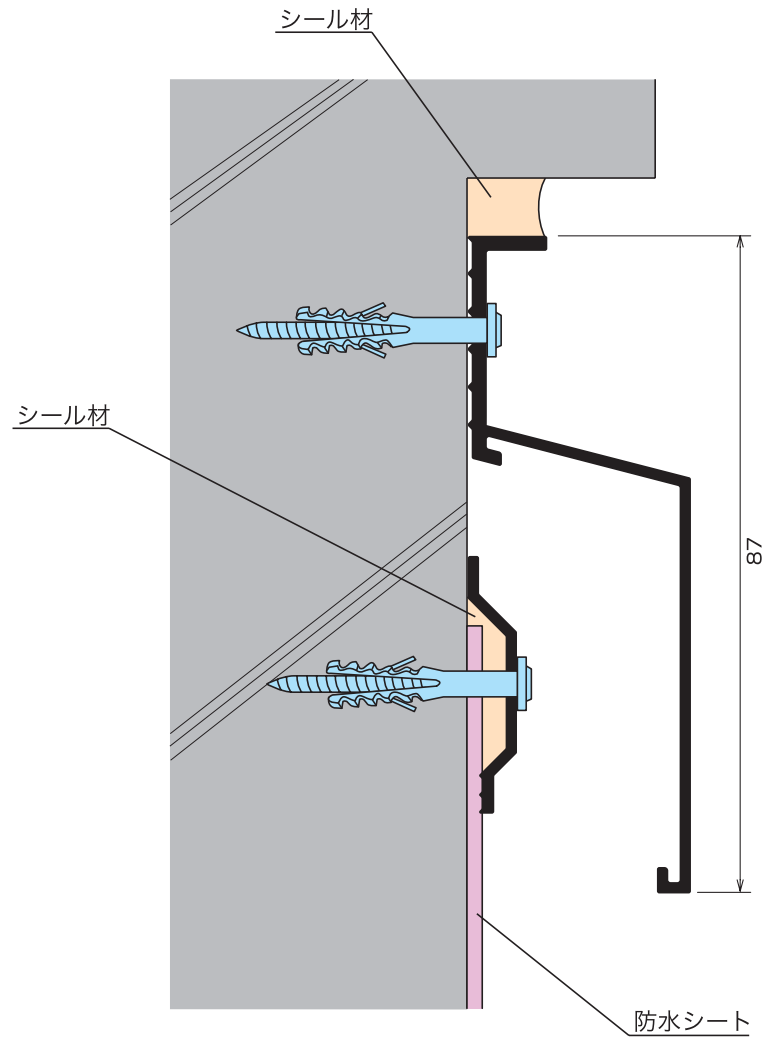
TA-201納まり図
