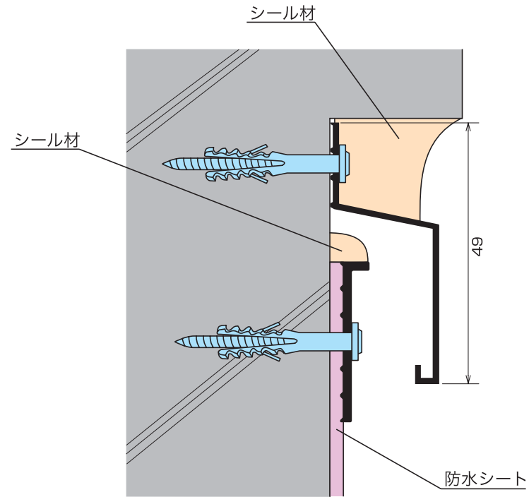
TA-209納まり図
