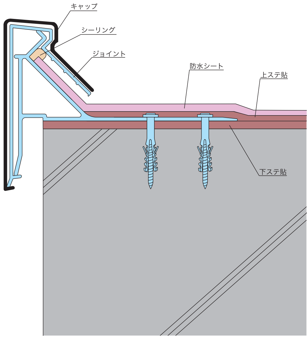
TA-250セット納まり図
