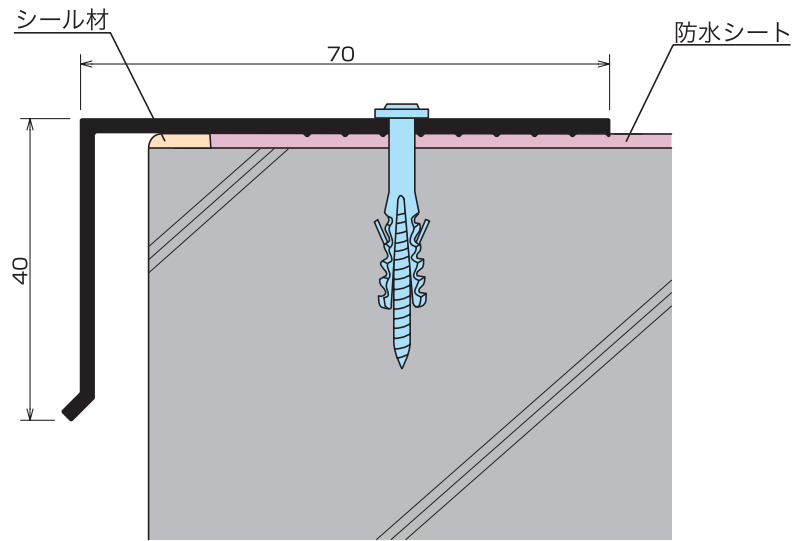
TA-70納まり図
