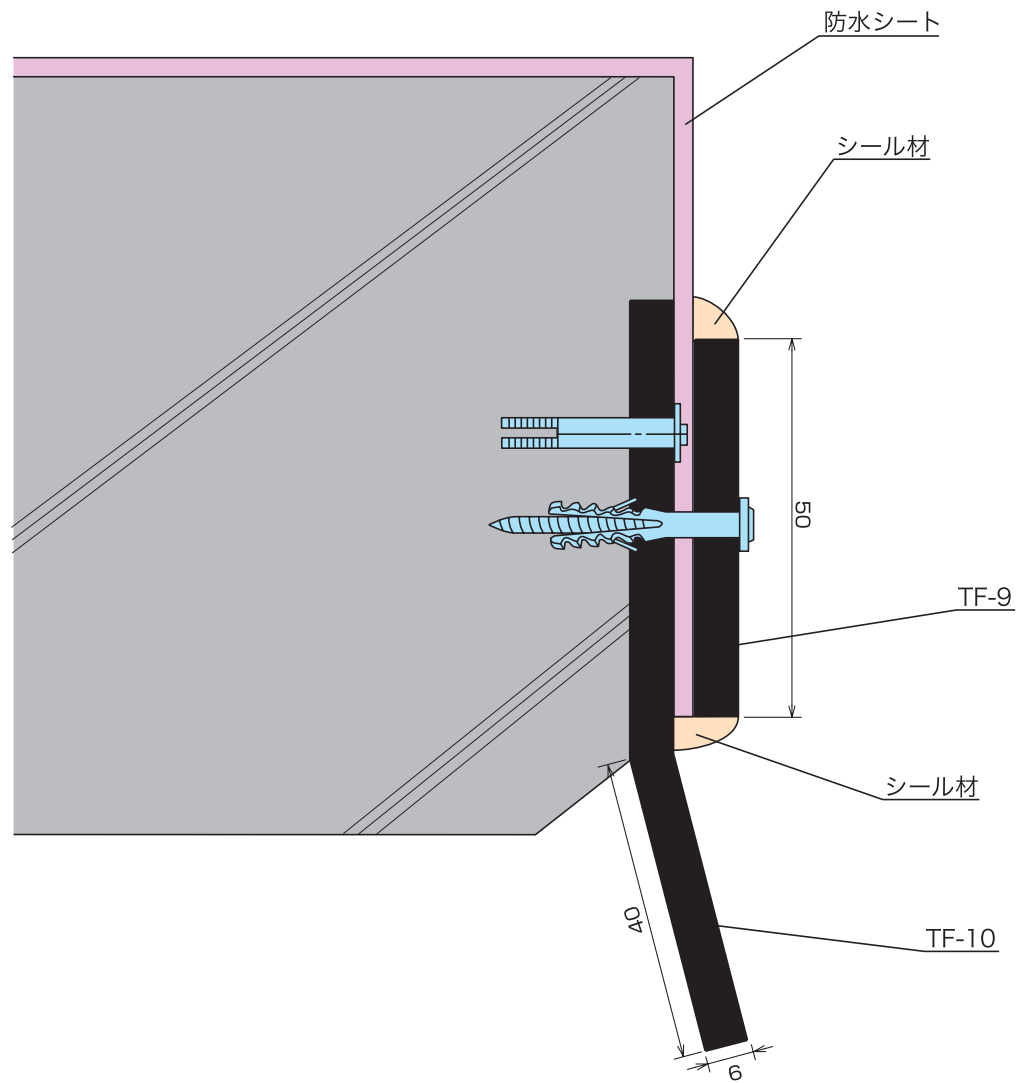
TF-9・TF-10納まり図
